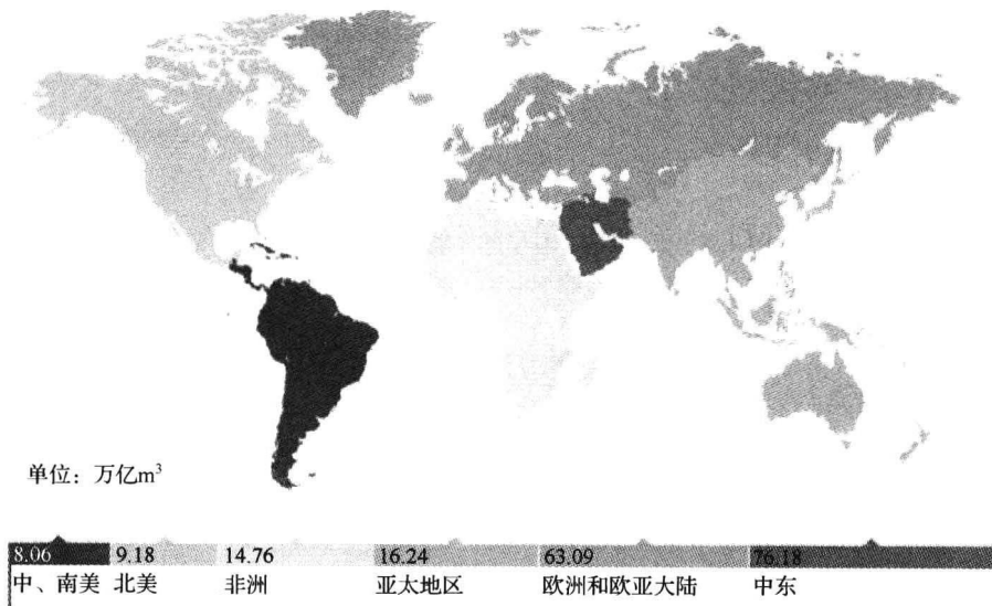
图 1.3 2009 年全球天然气探明储量分布
