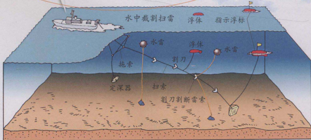
扫雷舰
