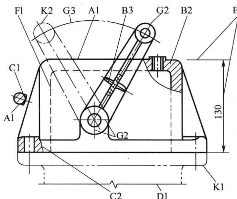
图 1-3 线型应用示例
