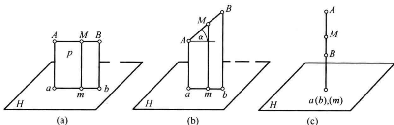
图 1-6 直线的投影特性
