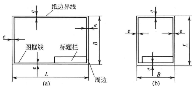
图 1-2 不留装订边图样的图框格式
