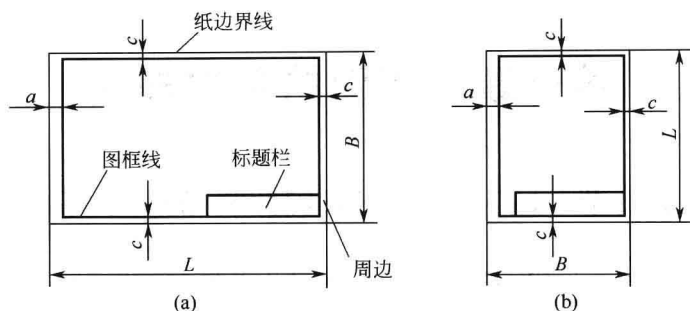
图 1-1 留有装订边图样的图框格式
