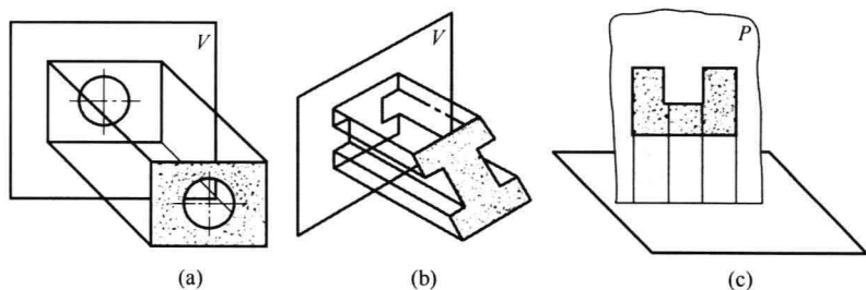
图 1-7 平面的投影特性
