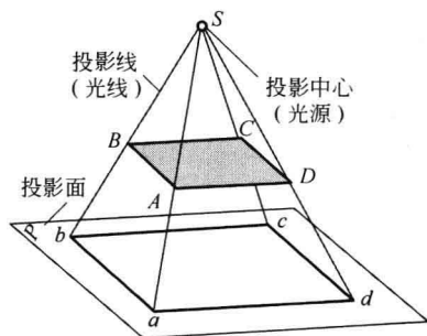
图 1-4 中心投影法
