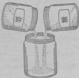
图 2-2 两种化合物相混和，但并未化合。
