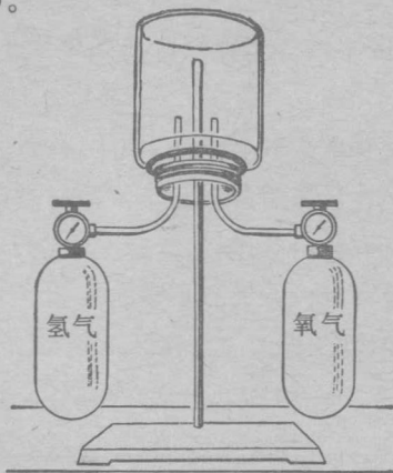
图 2-1 两种元素相混和，没有化合。
