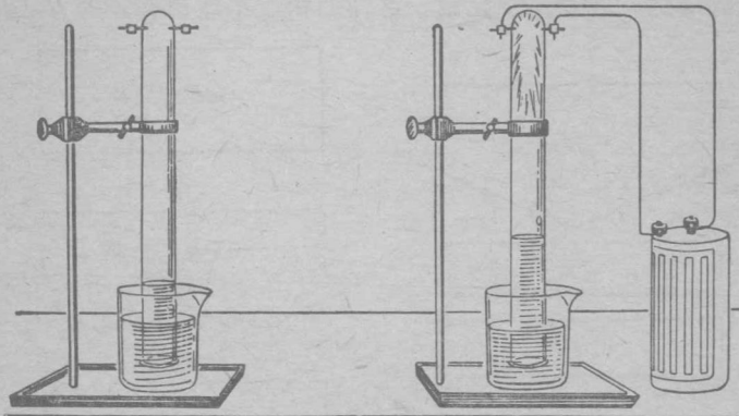
图 1-3 在这个实验里，我们做与图 1-2 相反的工作，在这里是把氢和氧化合成为水，这也是一种化学变化。
