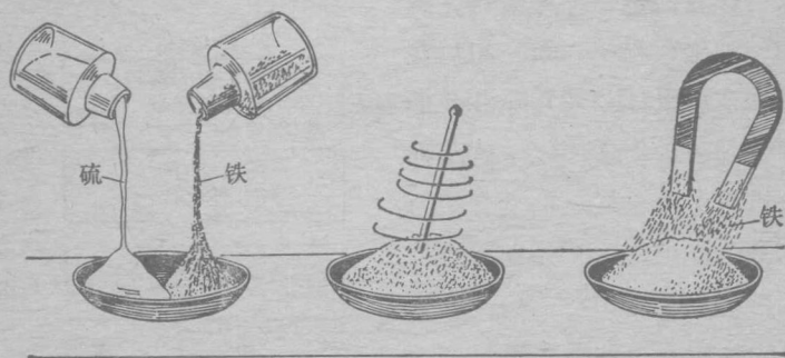
图 2-5 混和物的两种成分是很容易用磁铁分开的。可以用这个方法把铁从镍中分离出来吗？
