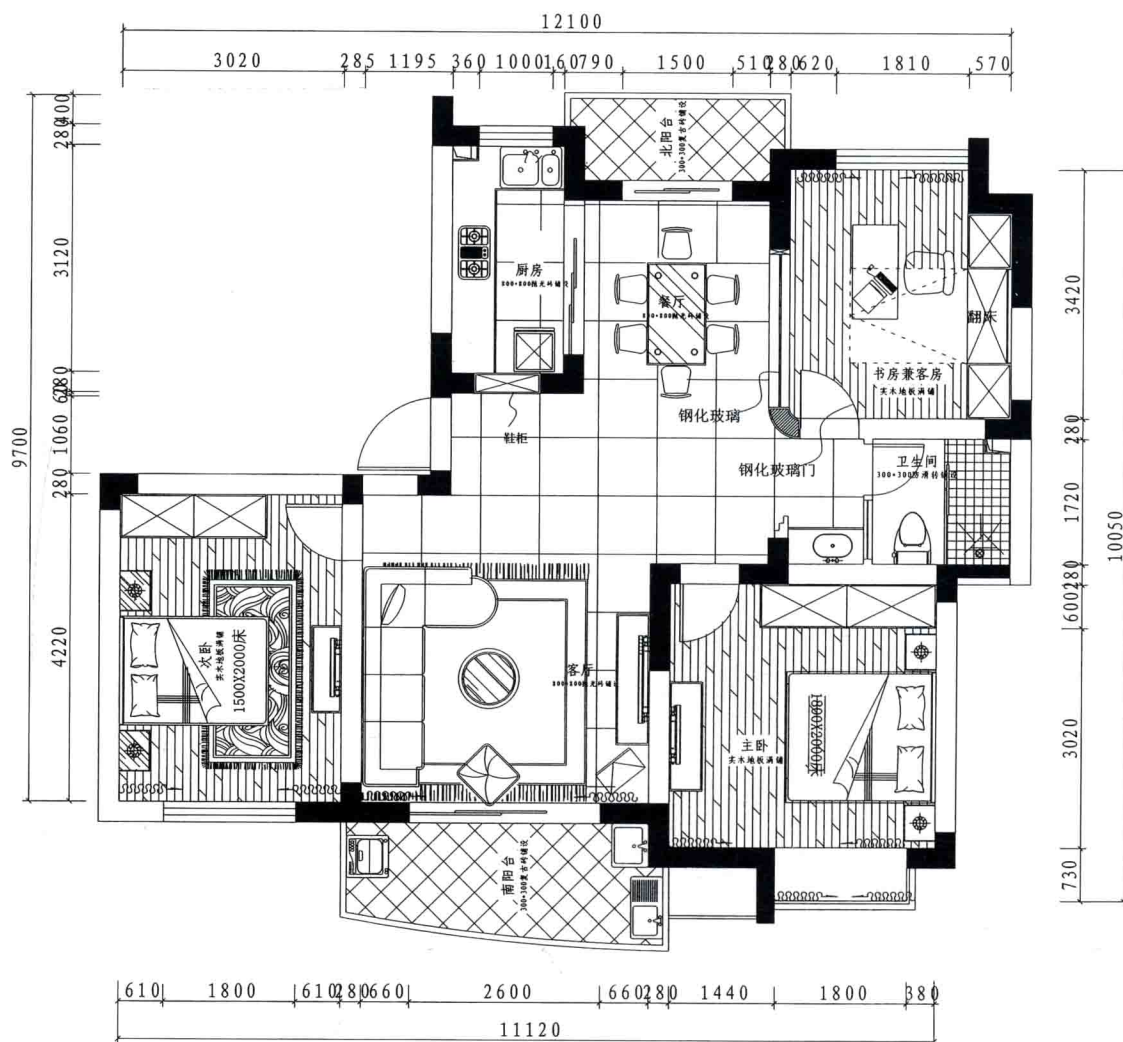
平面布置图
