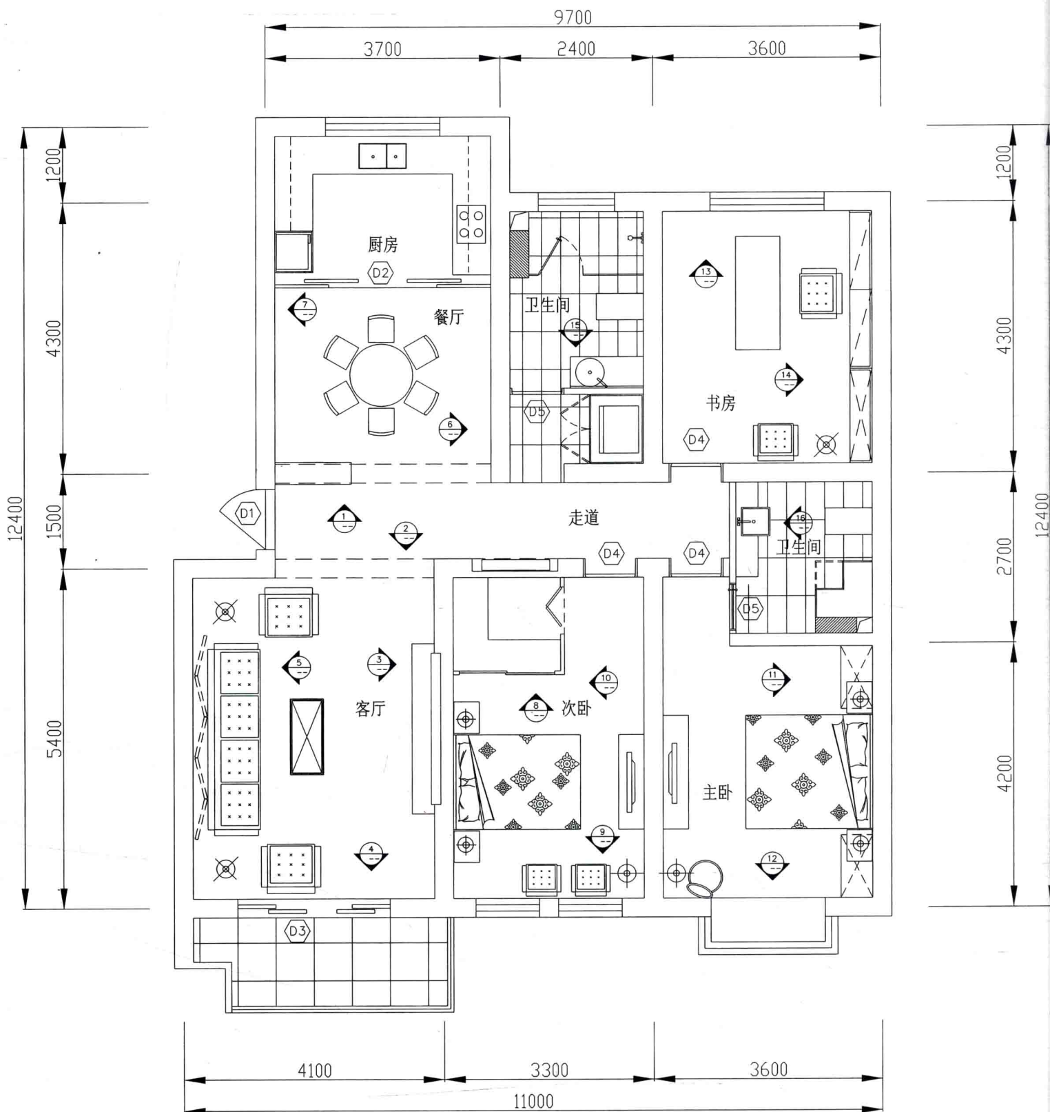
平面布置图
