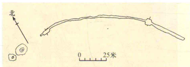
阿克色皮力古城平面图
