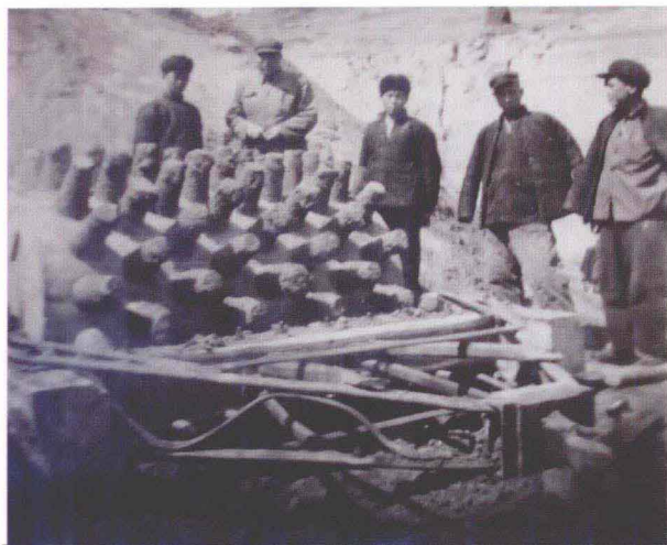
技术创新，轧实 坝体使用的羊角碾
