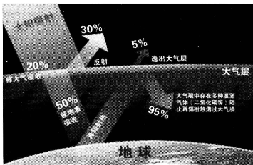
图 1-1 温室效应示意图（新华社发）
