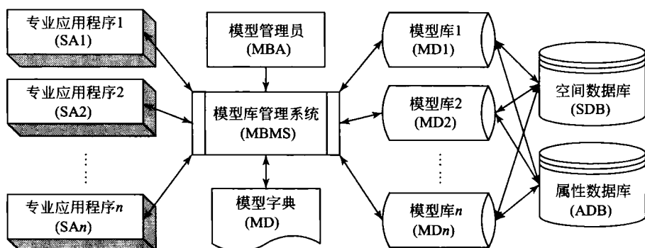
图 1-1 模型库系统运行图
