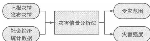
图 2-3 根据上报数据和发布数据评估洪涝灾情的流程
