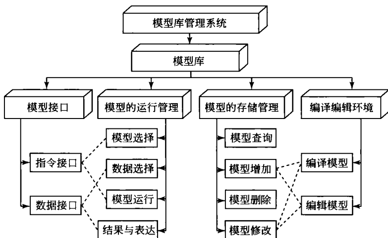
图 1-2 模型库管理系统组织方式
