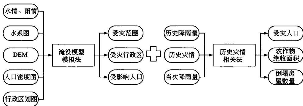
图 2-2 通过模拟和类比推测洪涝灾情的流程
