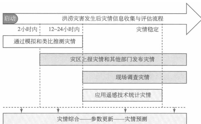
图 2-1 洪涝灾害灾情评估基本流程
