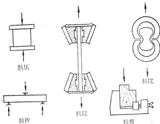
图 1-1 材料承受各种外力示意图
