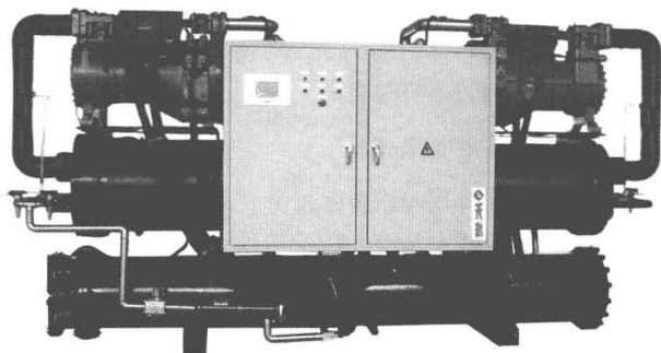
地源双机头螺杆机组
