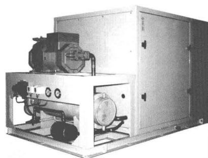
舰船组装式空调装置
