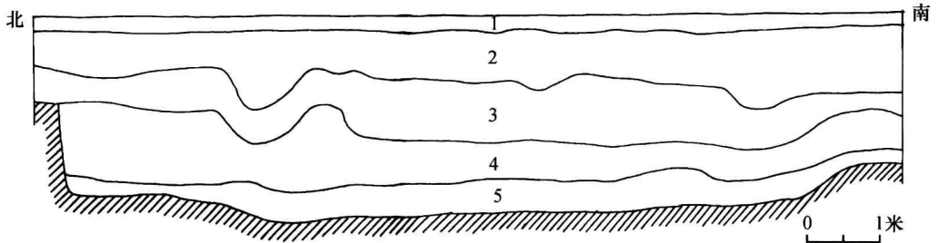
图4 T1015、T1115、T1215 东壁剖面图
