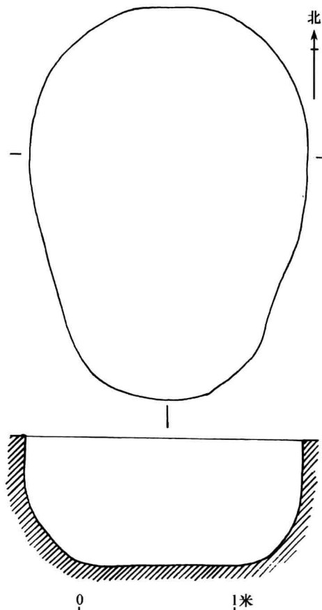
图5 H1平、剖面图
