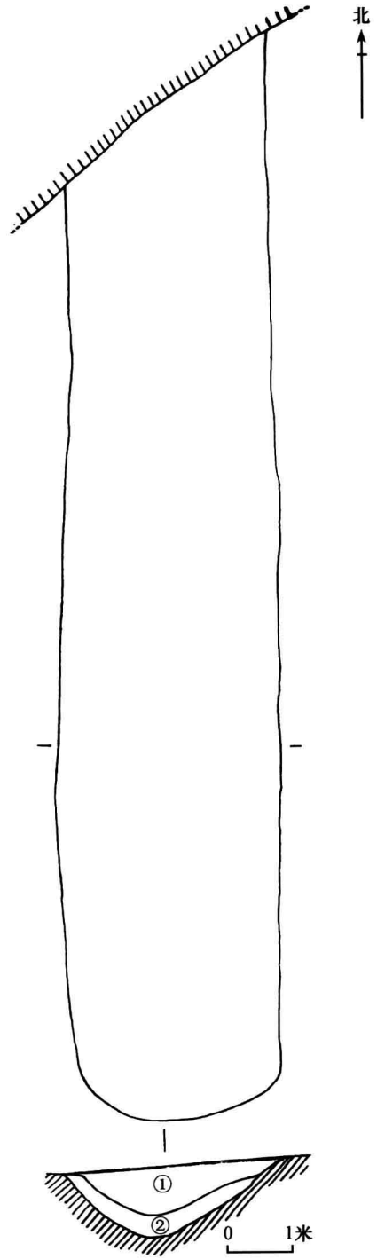
图 7 G1 平、剖面图
