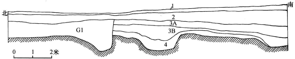
图3 T304、T404、T504 东壁剖面图
