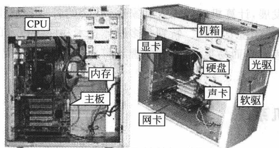
图 1-2 计算机机箱内部的结构
