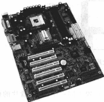
图 1-5 标准 ATX 结构的 Pentium 4 主板
