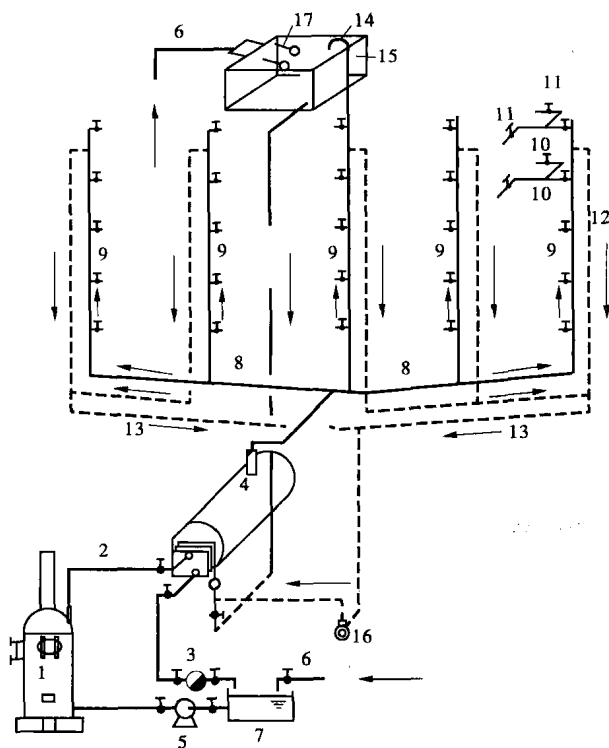
1—锅炉;2—热媒上升管(蒸汽管);3—热媒下降管(凝结水管);4—水加热器;5—给水泵(凝结水泵); 6—给水管;7—给水箱(凝结水箱);8—配水干管;9—配水立管;10—配水支管;11—配水龙头;12—回水立管; 13—回水干管;14—透气管;15—冷水箱;16—循环水泵;17—浮球阀
