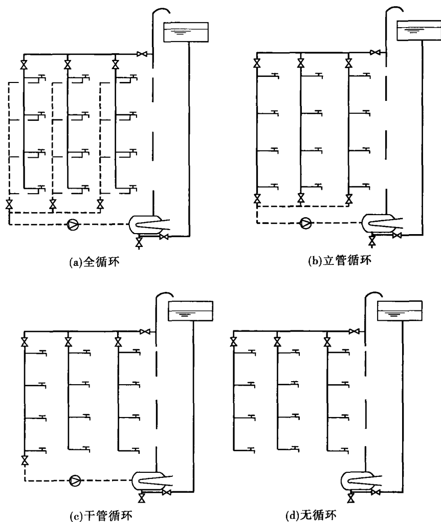
图 1-10 热水管网的循环方式
