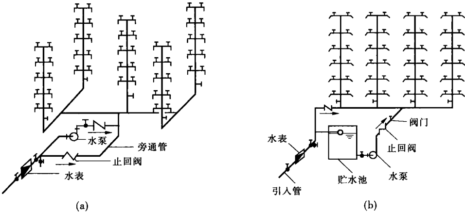
图 1-4 单设水泵的给水方式
