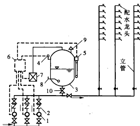
1—水泵;2—止回阀;3—气压水罐;4—压力信号器;5—液位信号器; 6—控制器;7—补气装置;8—排气阀;9—安全阀;10—阀门
