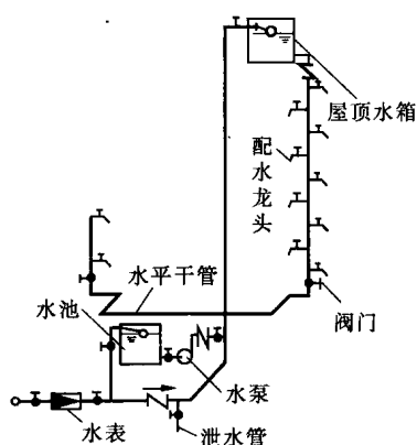
图 1-5 设贮水池、水泵和水箱的给水方式
