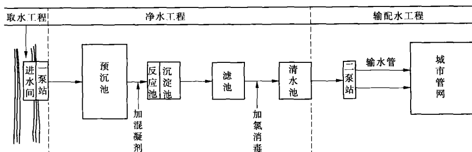
图 1-11 以地面水为水源的城市给水系统图式
