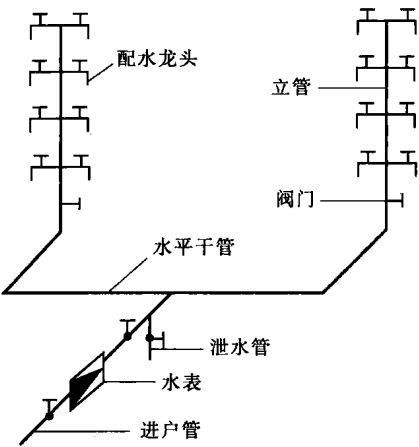
图 1-2 室外管网直接给水方式
