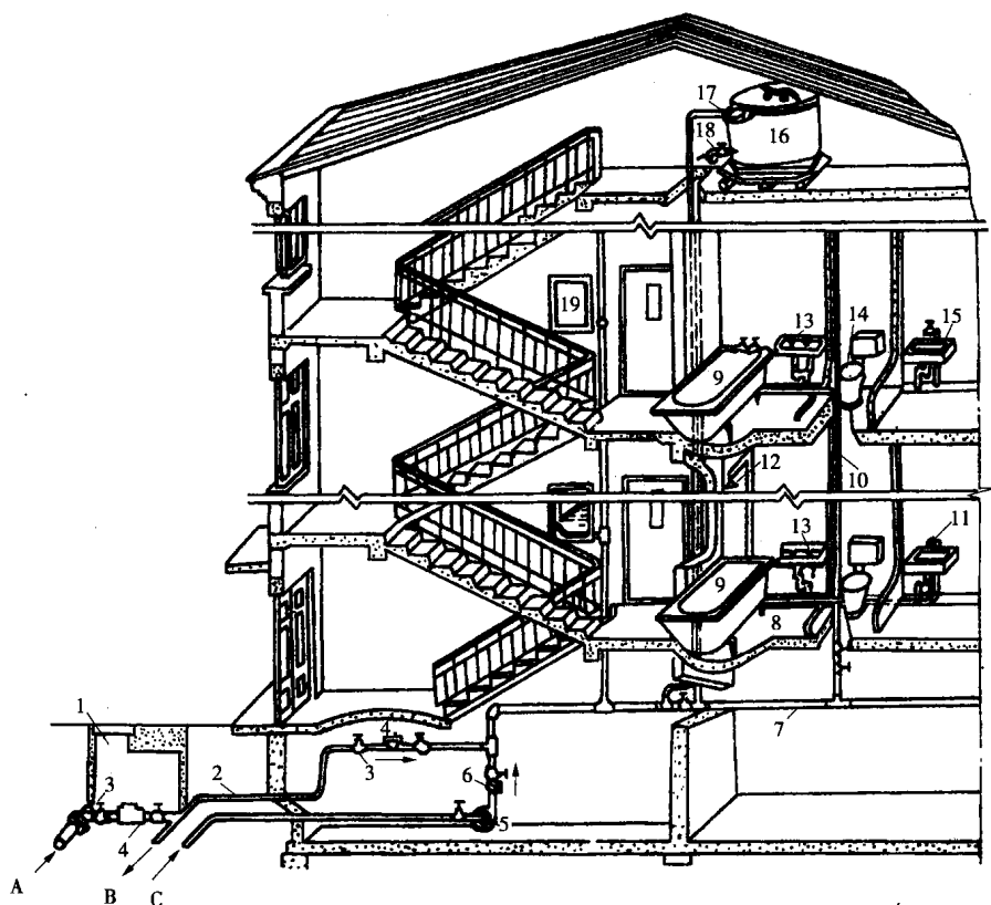
1—阀门井;2—引入管;3—闸阀;4—水表;5—水泵;6—止回阀;7—干管;8—支管;9—浴缸;10—立管; 11—水龙头;12—淋浴器;13—洗脸盆;14—大便器;15—洗涤盆;16—水箱;17—进水管;18—出水管; 19—消火栓;A—从室外管网进水;B—入贮水池;C—来自贮水池
