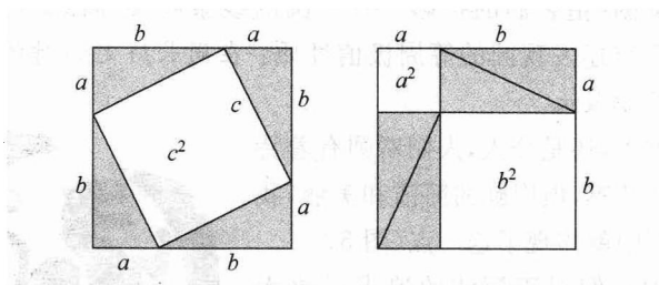
图7 勾股(毕达哥拉斯)定理的证明
