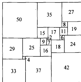
图 14 21 阶完美正方形
