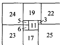
10阶完美矩形
