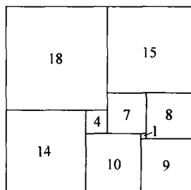
9阶完美矩形
