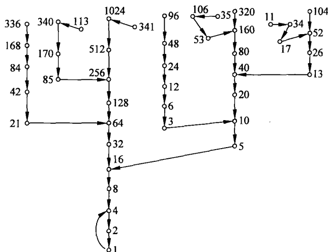
图 15 某些数经 3x+1 运算的路径
