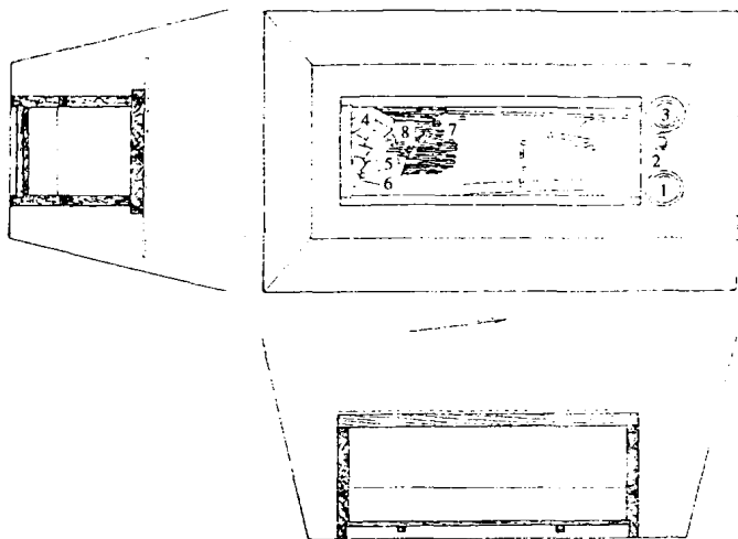
图二 M15 平、剖面图 (1/10)
