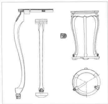
明 三腿香几结构图
