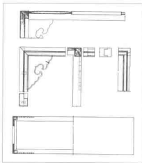
明 琴几结构图
