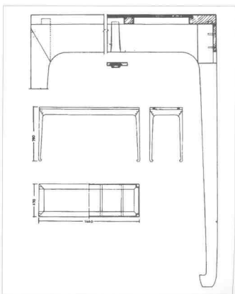
明 琴几结构图
