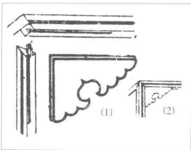
明 琴几托角榫结构图
