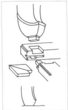
明托泥桌几结构图
