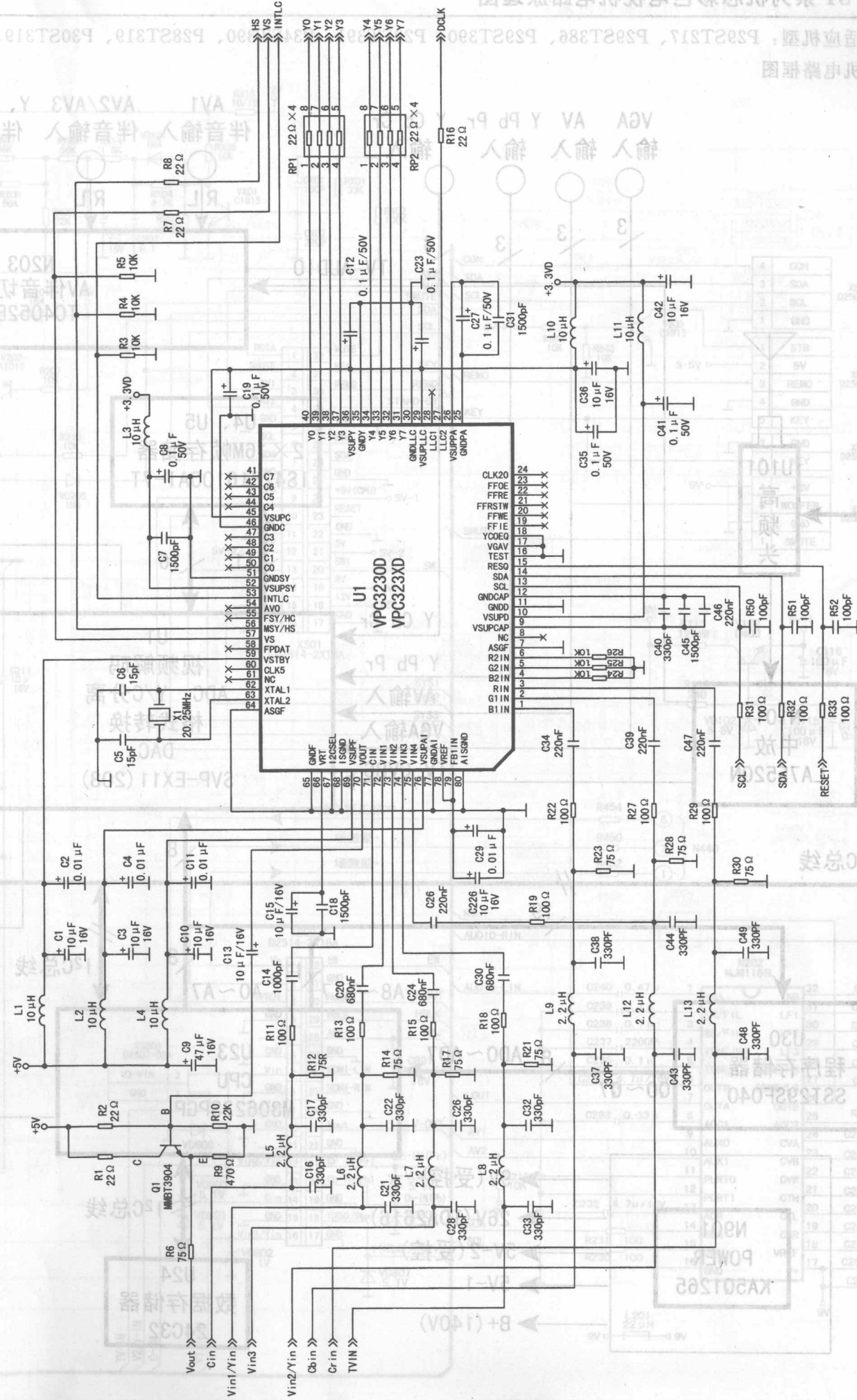
(11) TV 视频解码-数字分量输出电路
