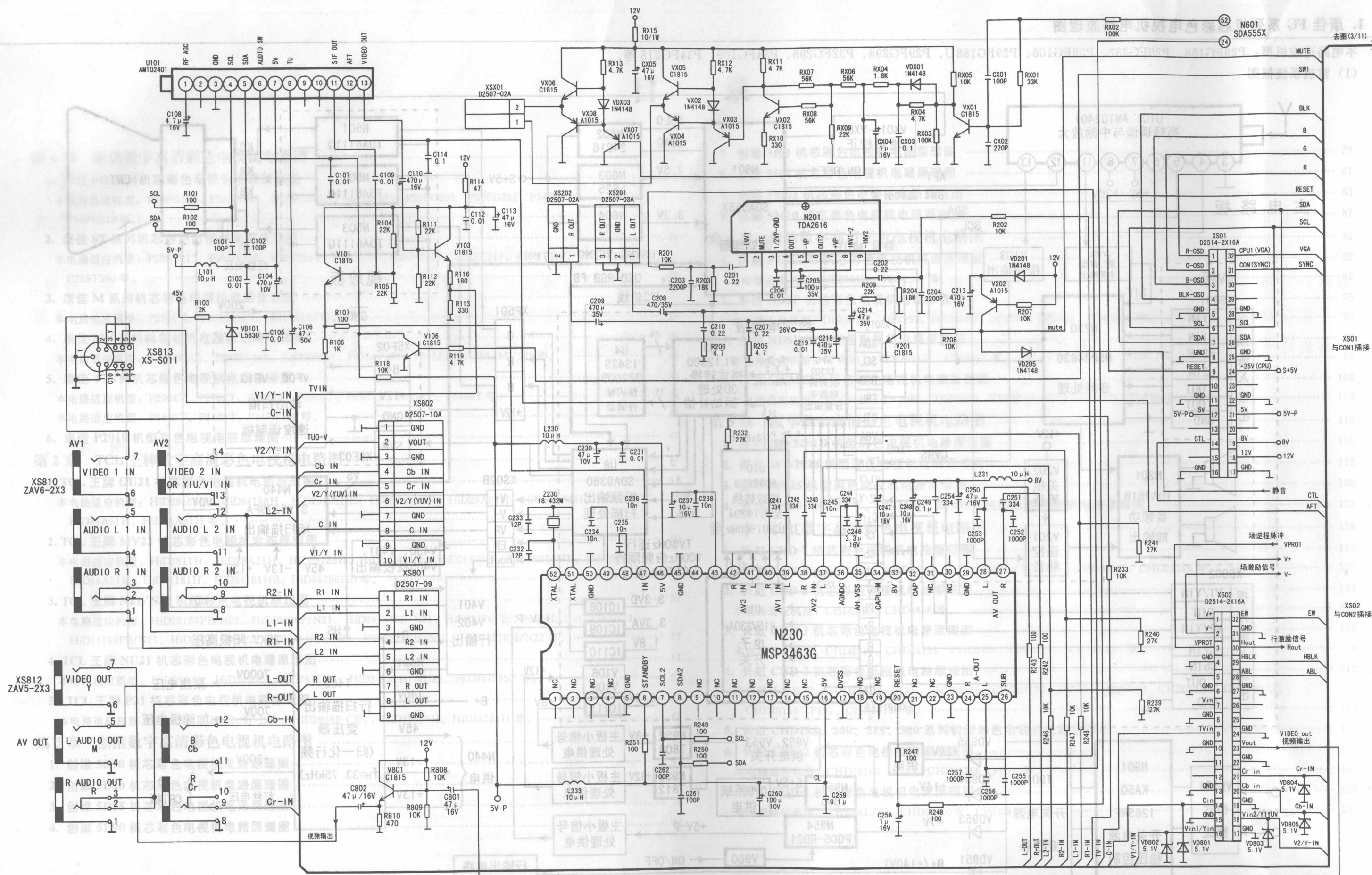
(2) 主板 (高频头含中频处理、伴音处理、地磁校正电路)
