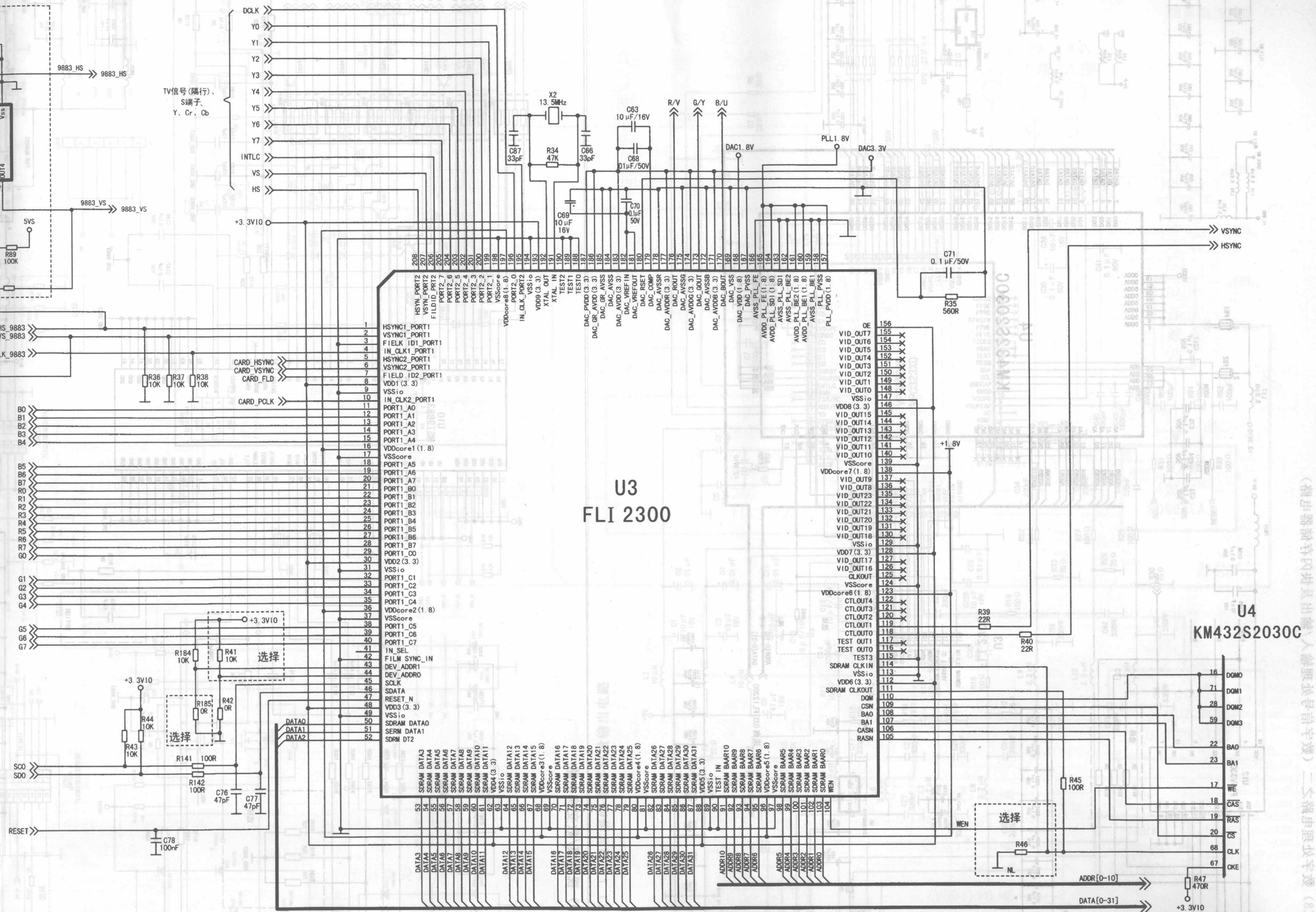
(7) 数字处理电路之一 (数字信号处理输入/输出及快闪存储器电路)
