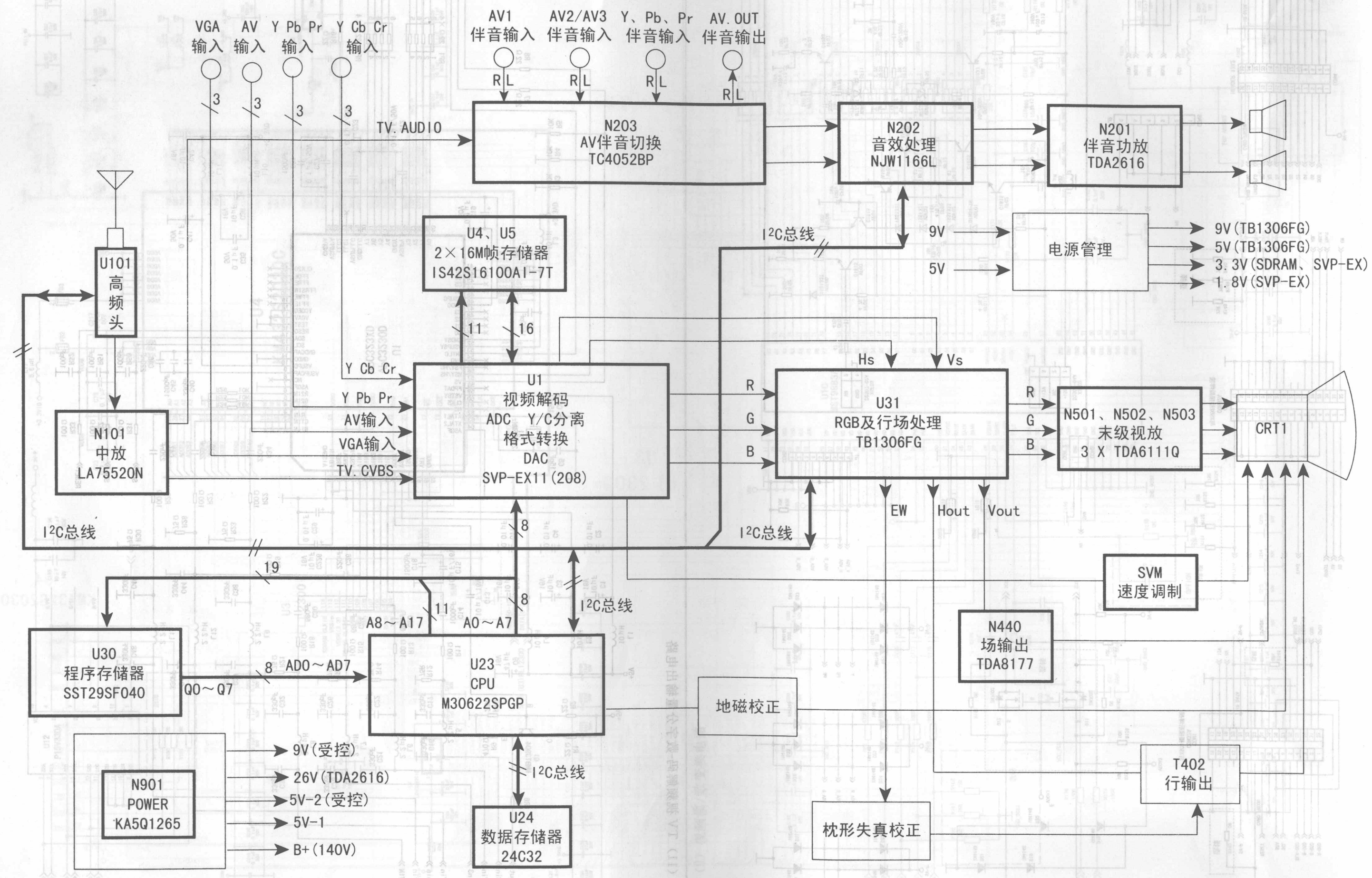
(1) 整机电路框图
