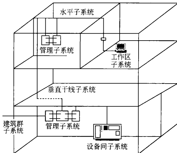
图 1.3 综合布线系统
