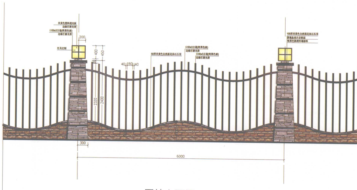
围墙立面图
