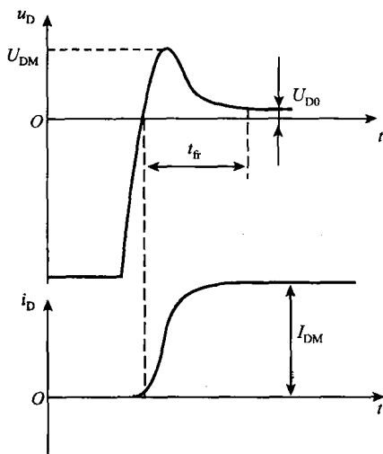
图 1-4 大功率二极管的开通过程
