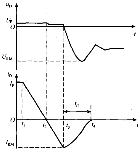
图 1-5 大功率二极管的关断过程
