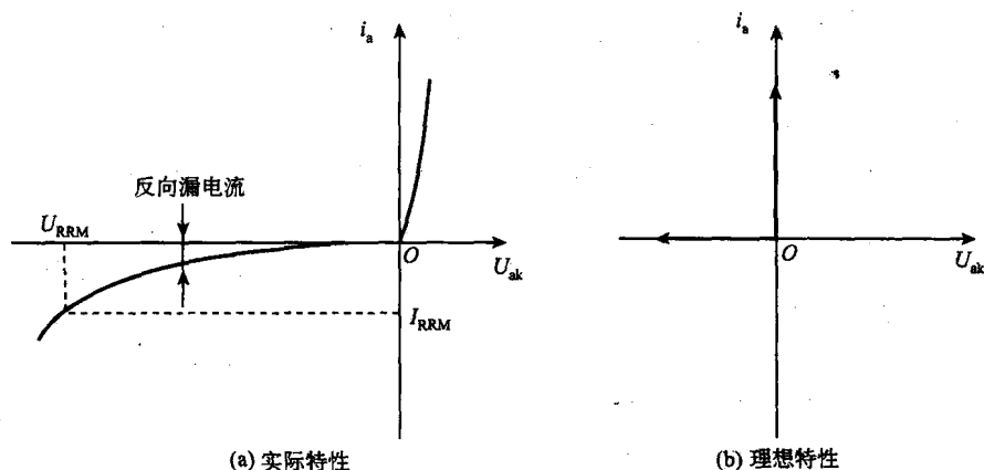
图 1-3 大功率二极管的伏安特性
