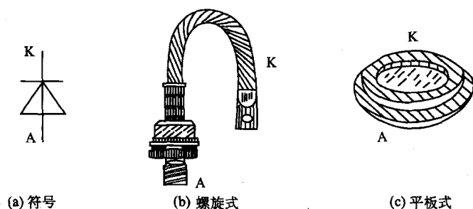
图 1-2 大功率二极管
