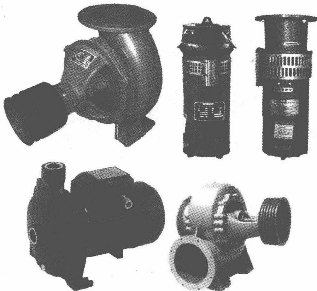
图 1-1 农用泵外形
