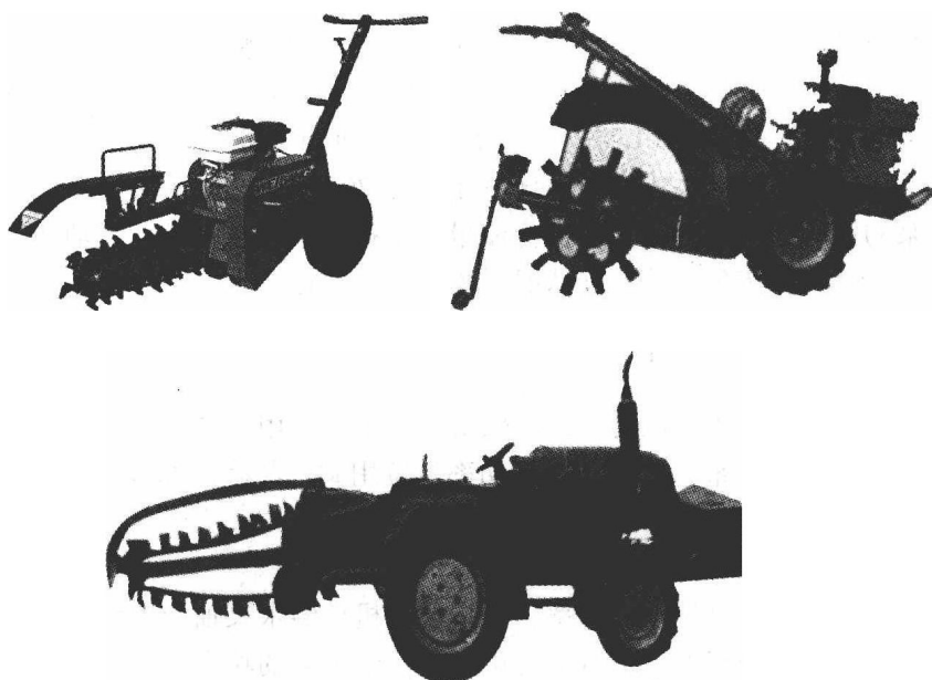
图 1-5 开沟机外形
