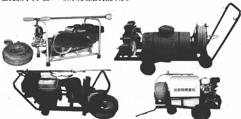
图 1-3 喷灌机械外形
