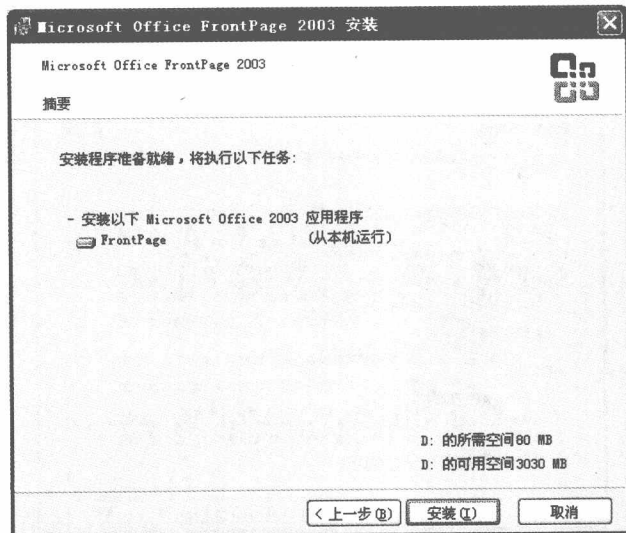
图 1.2.6 “摘要”对话框
