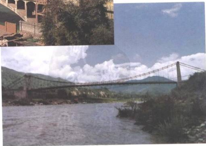
柔式吊桥
