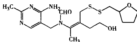
呋喃硫胺
