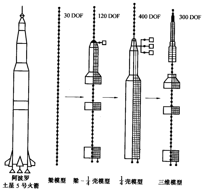
图 0.3 阿波罗土星 5 号的各种计算模型
