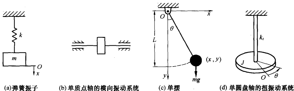
图 1.1 单自由度系统
