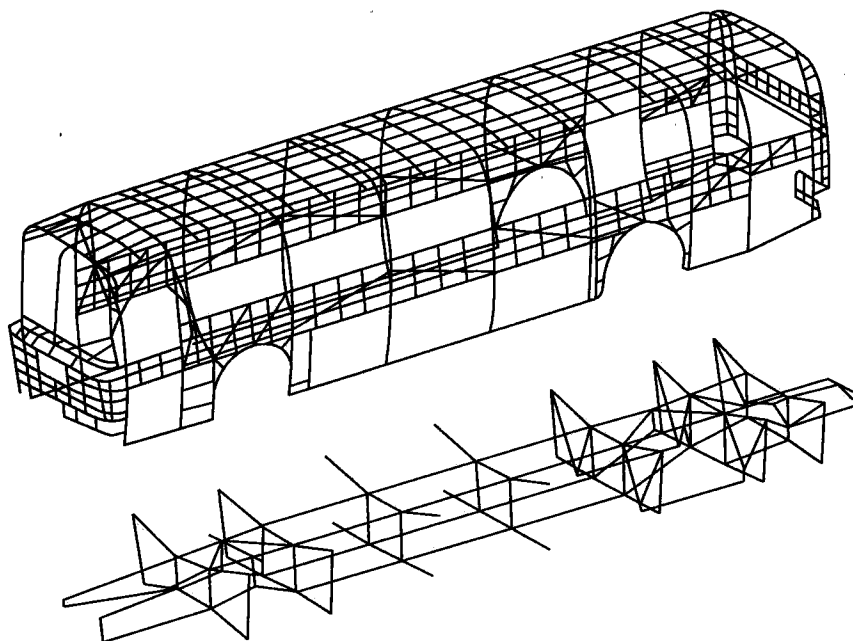
图 0.4 大型客车的车身和底盘的有限元模型
