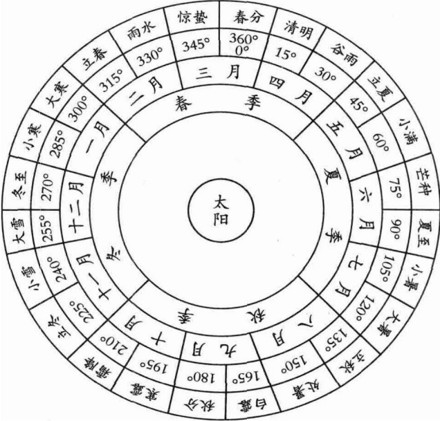
黄道与二十四个节气
