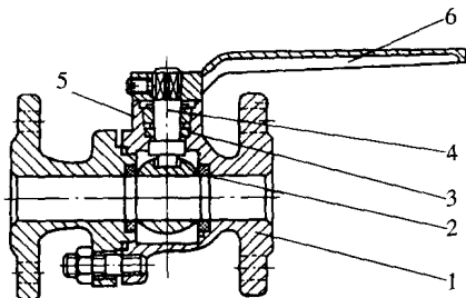
图 1-5 球阀
