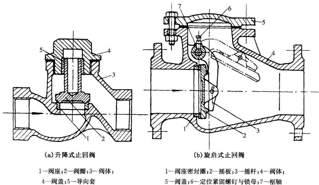
图 1-8 止回阀
