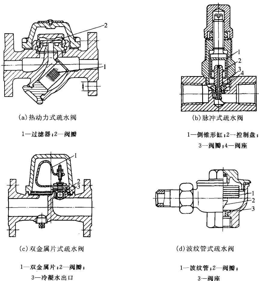
图 1-7 疏水阀
