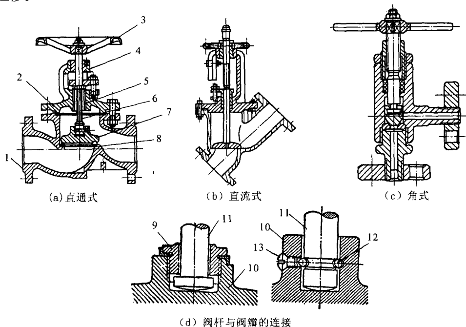
图 1-1 截止阀
