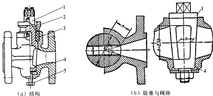
图 1-2 旋塞阀(考克)
