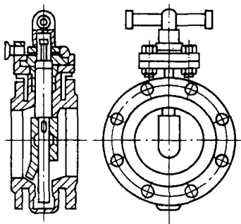
图 1-3 蝶阀
