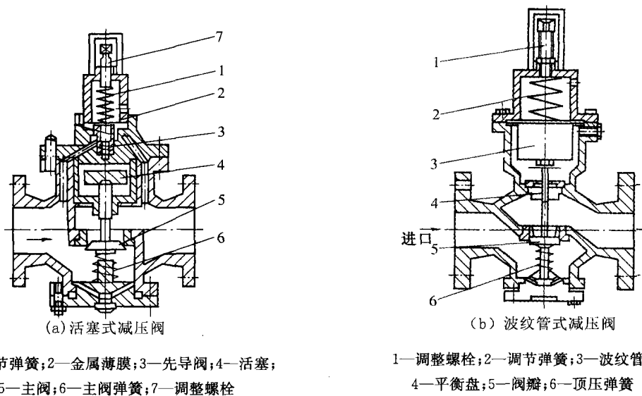
图 1-6 减压阀
