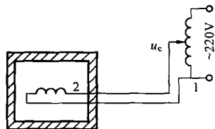
图 1-3 炉温开环控制系统
