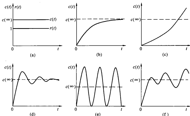
图 1-9 系统单位阶跃响应曲线
