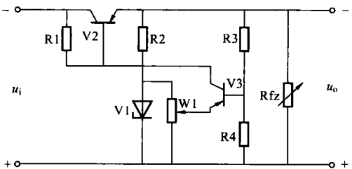
图 1-15 习题 1-10 的晶体管直流稳压电路原理图
