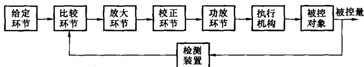
图 1-7 闭环系统组成方框图
