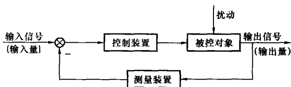
图 1-4 闭环控制示意图
