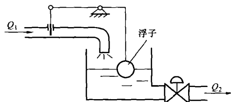
图 1-10 习题 1-5 的水位自动控制系统示意图
