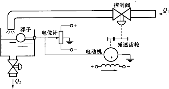
图 1-11 习题 1-6 的液位自动 控制系统的示意图
