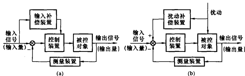
图 1-6 复合控制示意图
