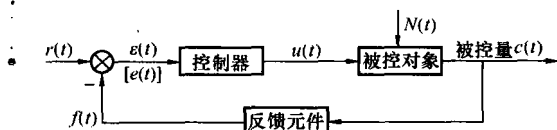
图 1-8 简化的闭环系统组成方框图
