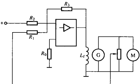
图 1-14 习题 1-9 的电压负反馈转速 自动控制系统的部分原理图
