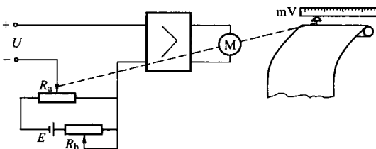
图 1-13 习题 1-8 的自动平衡仪表示意图
