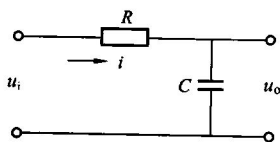
图 2-1 RC 无源网络
