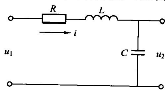
图 2-2 R、L、C 串联电路
