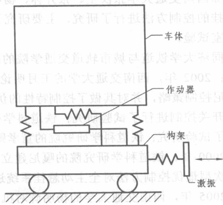
图 1.4 三自由度半车体试验模型
