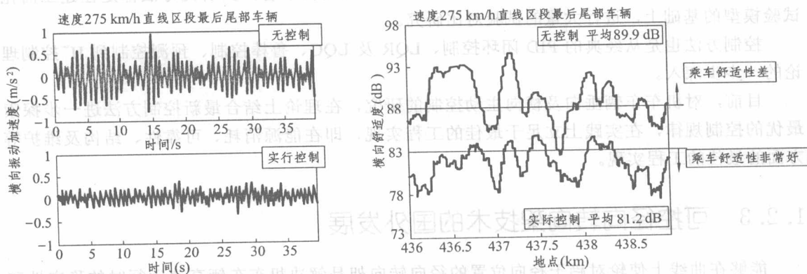
图 1.5 主动控制实测效果图
