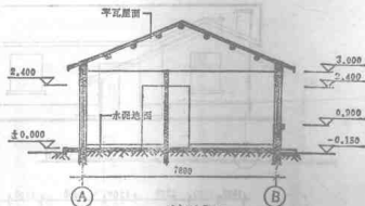
剖面图
