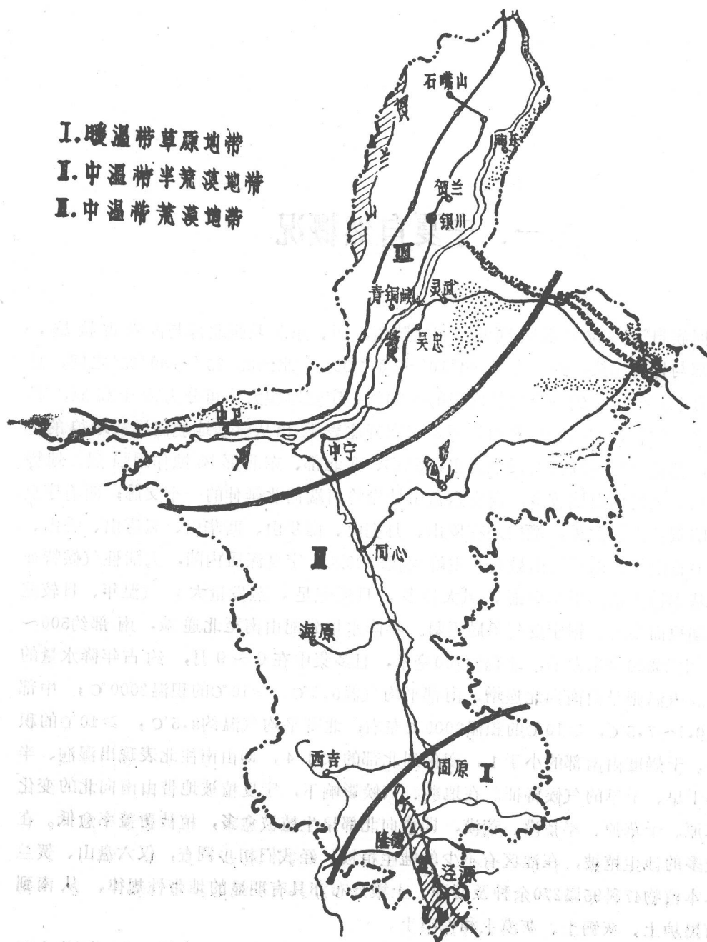
图1 宁夏回族自治区自然区划草图
