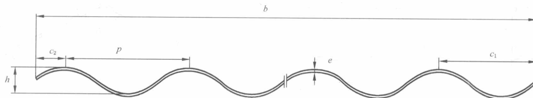
图1 大波瓦示意图
