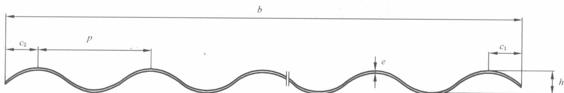
图2 中波瓦示意图
