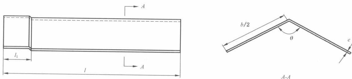
图4 脊瓦示意图
