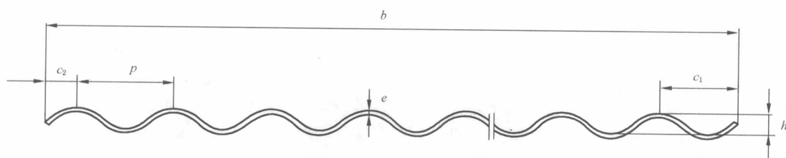
图3 小波瓦示意图
