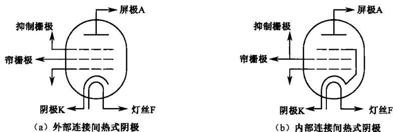
图 1-9 五极管的电路图形符号 (2)
