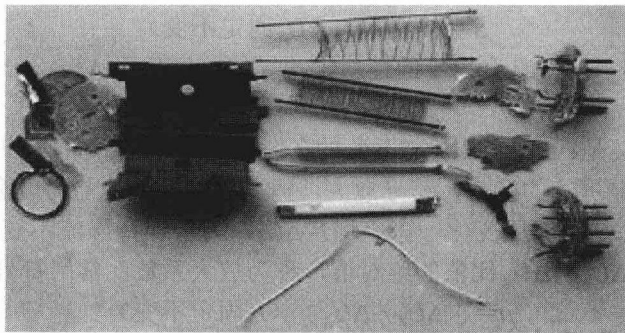
(m) 第十三步：拆散后的电子管照片
