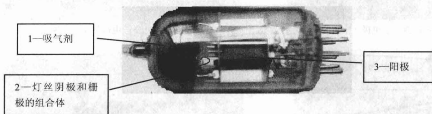
图 1-3 电子管 6N1
