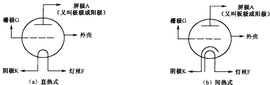
图 1-6 三极电子管的电路图形符号
