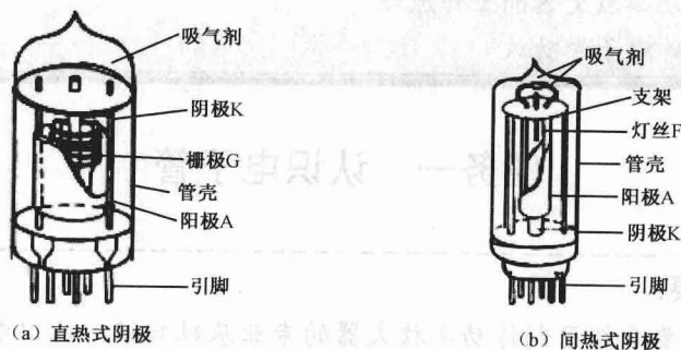
图 1-1 电子管外形
