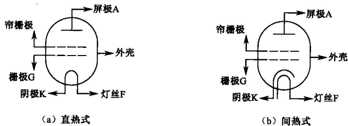
图 1-7 四极电子管的电路图形符号
