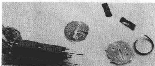
(e) 第五步：将固定电极的支架拆开后的电子管实物
