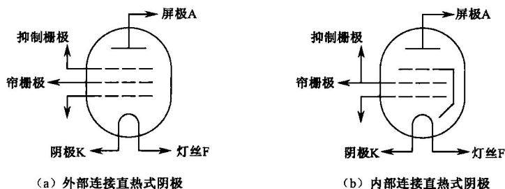
图 1-8 五极管的电路图形符号 (1)
