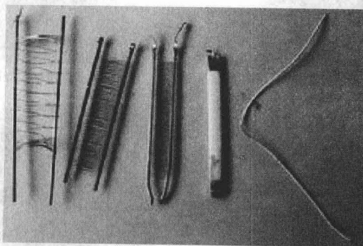
(l) 第十二步：电子管电极
