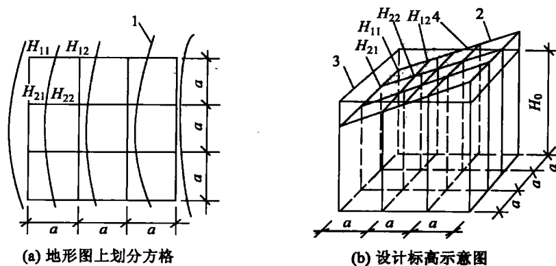
1—等高线;2—自然地坪;3—设计标高平面;4—自然地面与设计标高平面的交线(零线)
