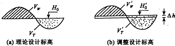
图 1.2.3 设计标高调整示意图
