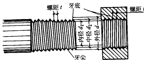
图 1-2 螺纹的主要尺寸
