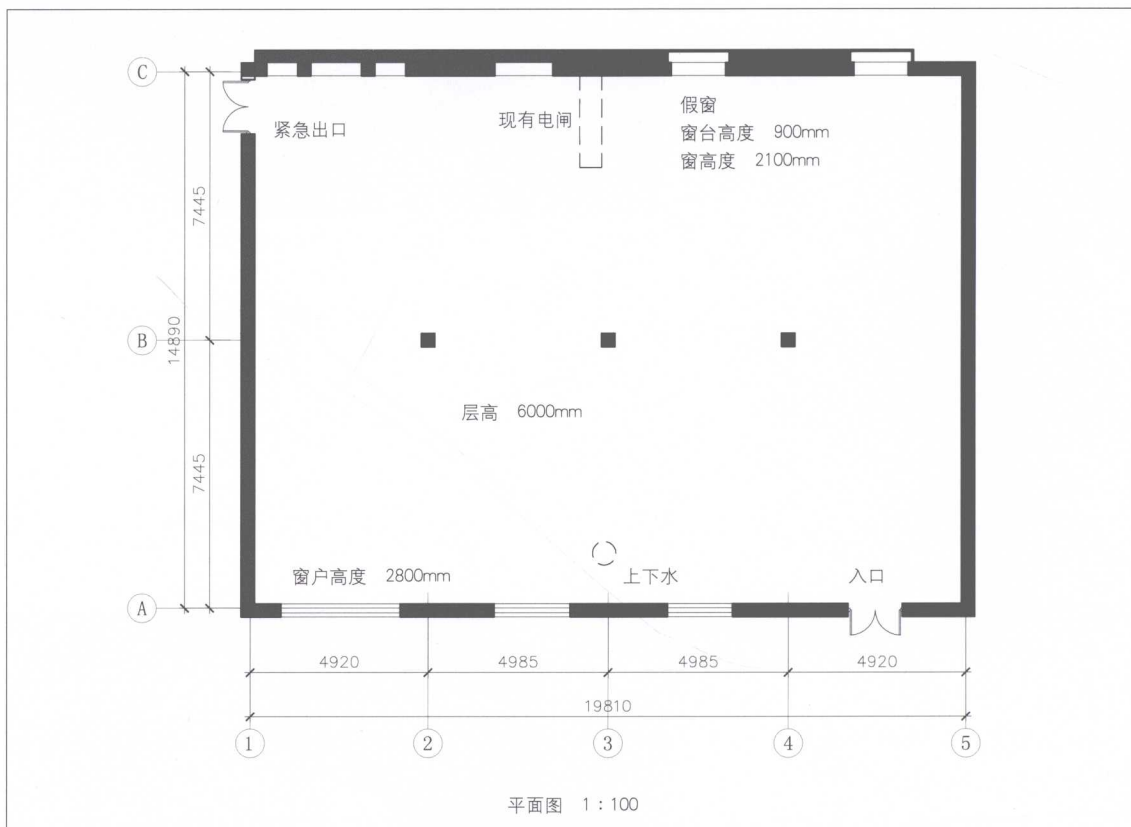
图2-1 原始平面图
