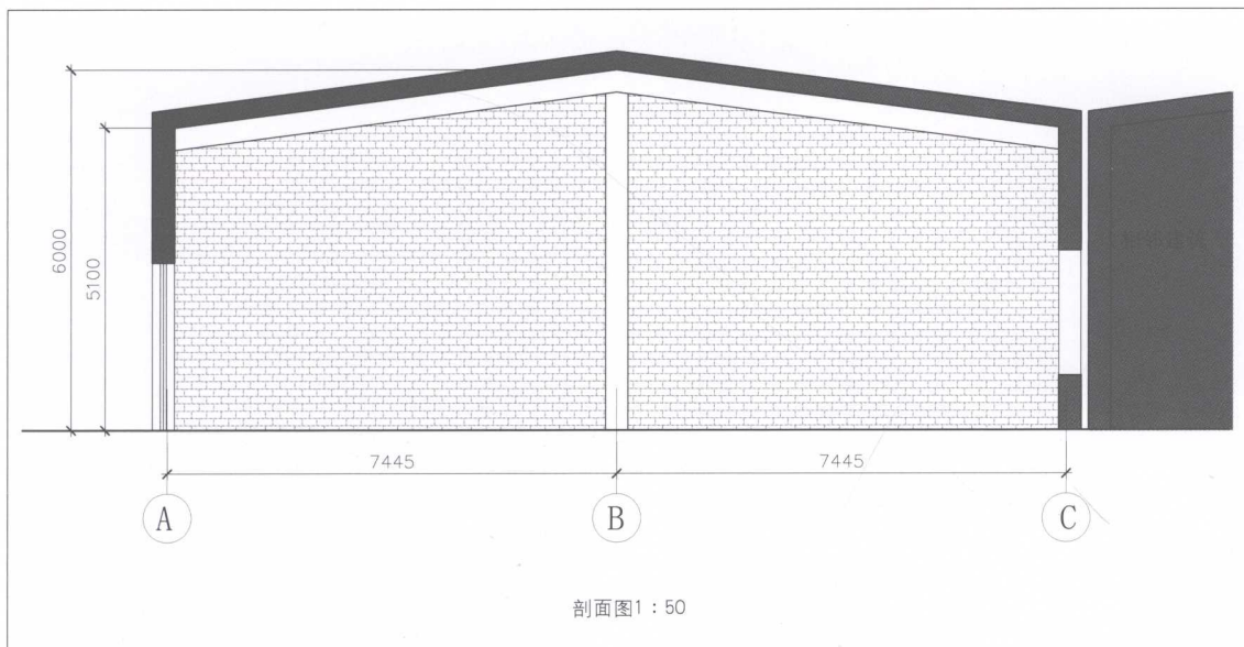
图2-2 原始剖面图
