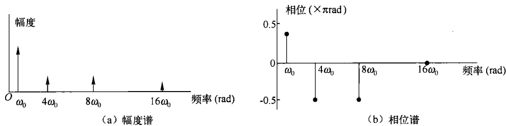
图 0-6 图 0-5(a) 所示信号的频谱
