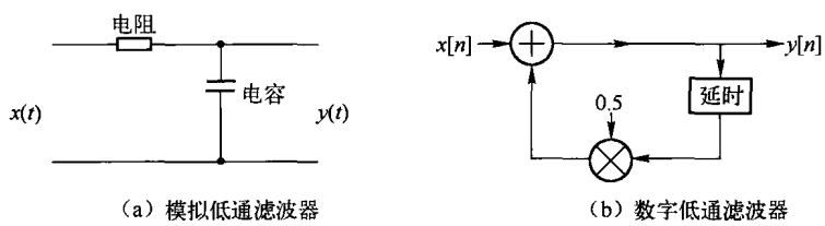
图 0-3 低通滤波器
