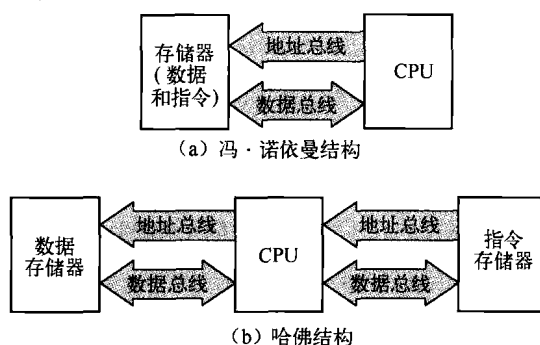
图 0-4 冯·诺依曼结构和哈佛结构
