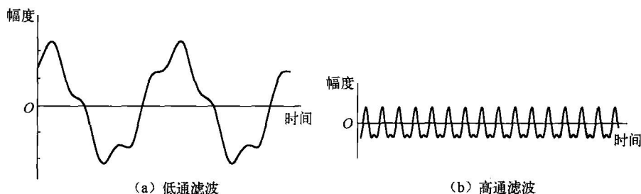
图 0-7 图 0-5(a)中的信号经过滤波器后的信号
