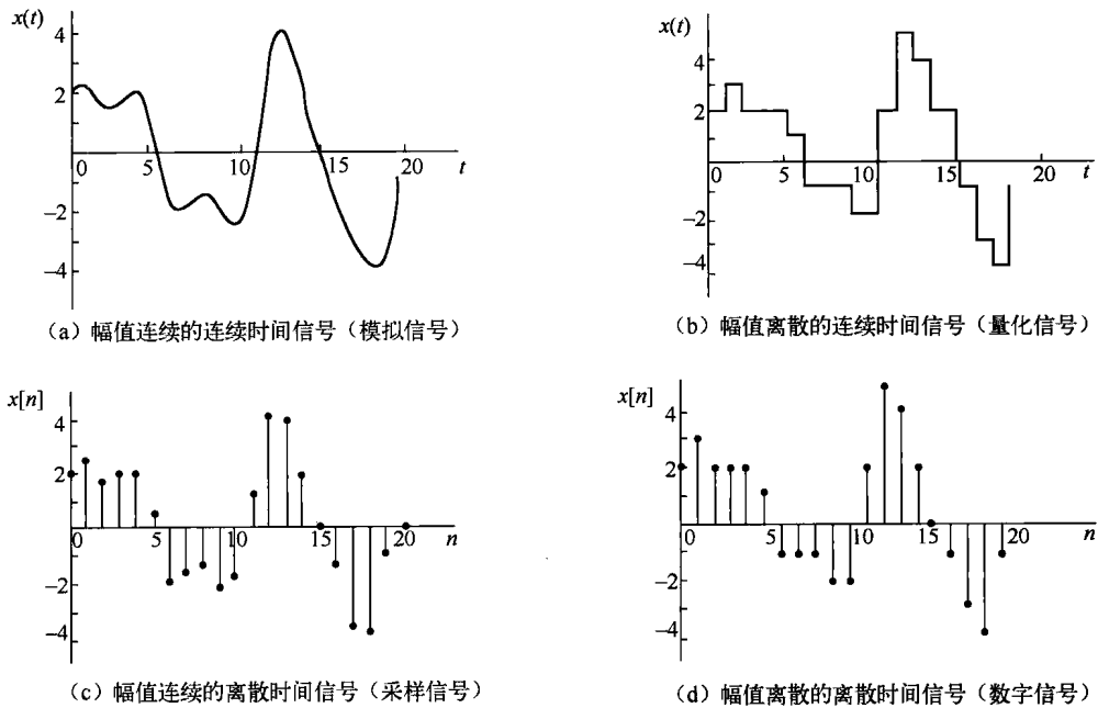
图 0-1 信号的分类
