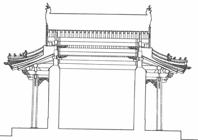
左翼王亭纵剖面图
