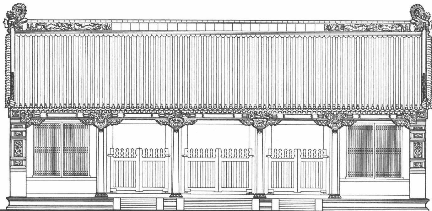
大清门正立面图
