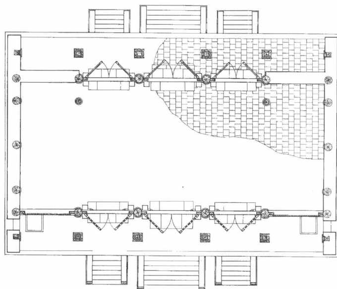
大清门平面图
