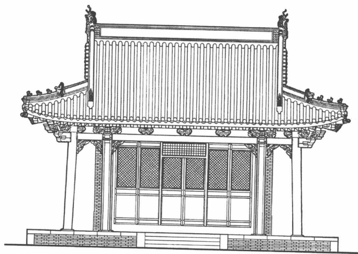
左翼王亭正立面图
