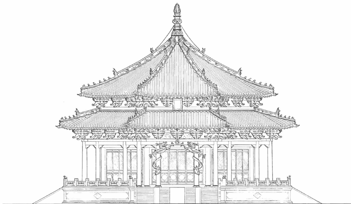
大政殿正立面图
