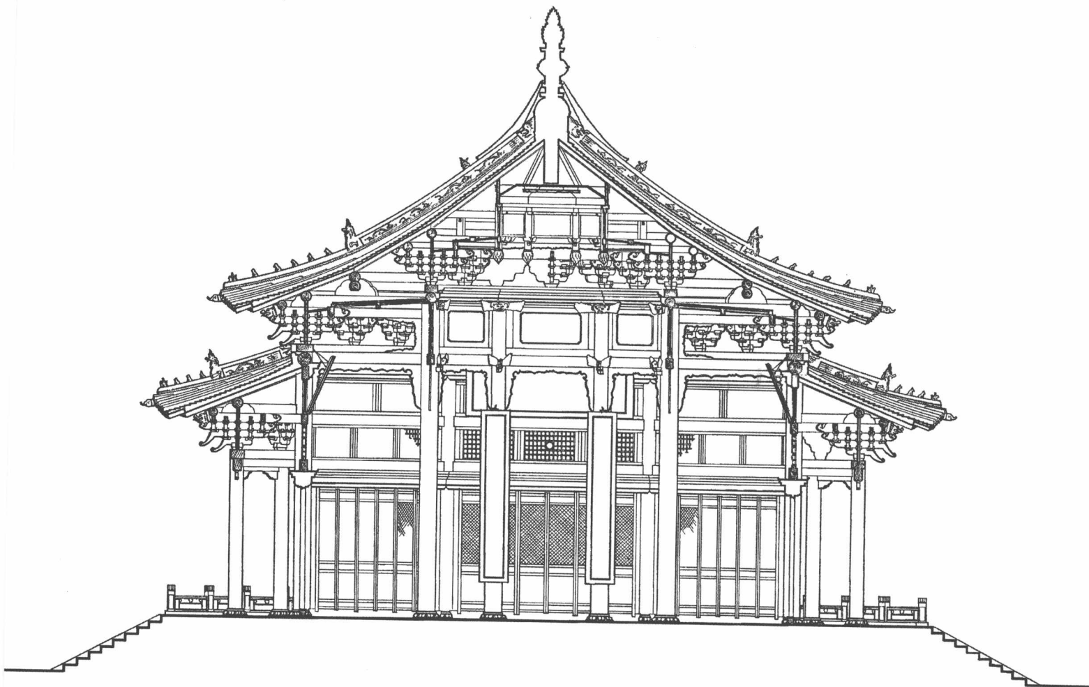
大政殿纵剖面图
