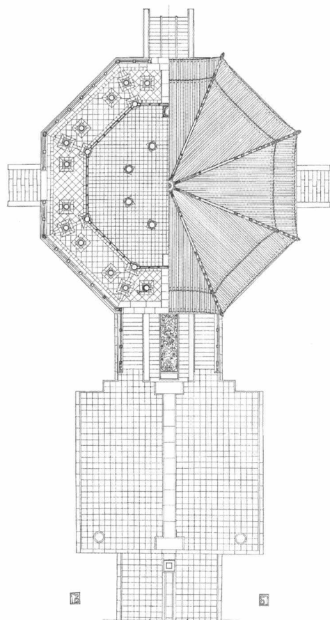
大政殿平面图
