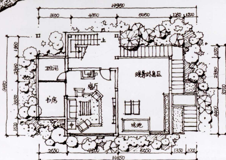
一层平面图
