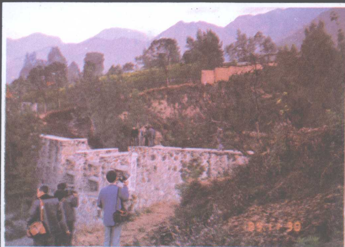
▼后山泥石流治理工程
