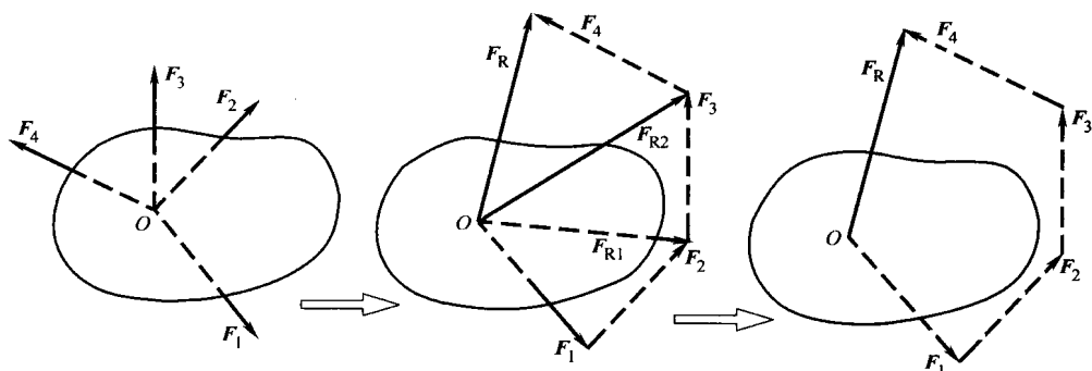
图 1-6 力的多边形法则
