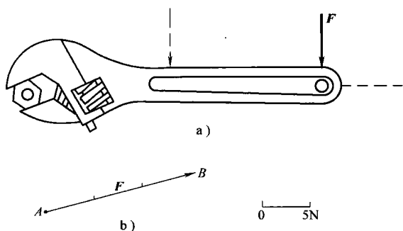
图 1-1 力的表示
