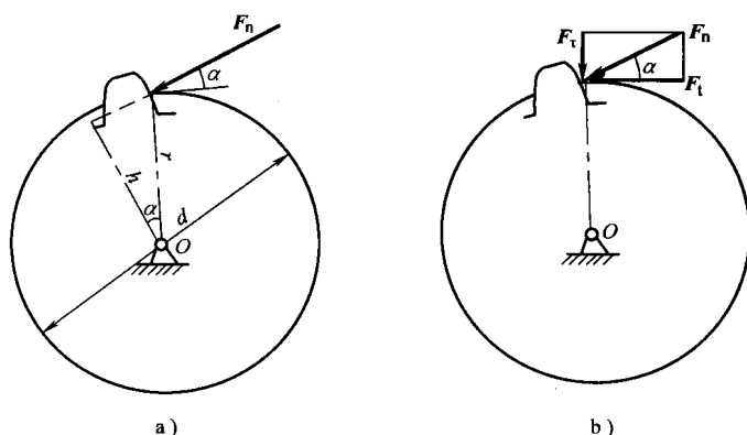
图 1-10 直齿圆柱齿轮力矩的计算
