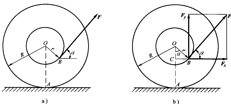
图 1-11 轮轴力矩
