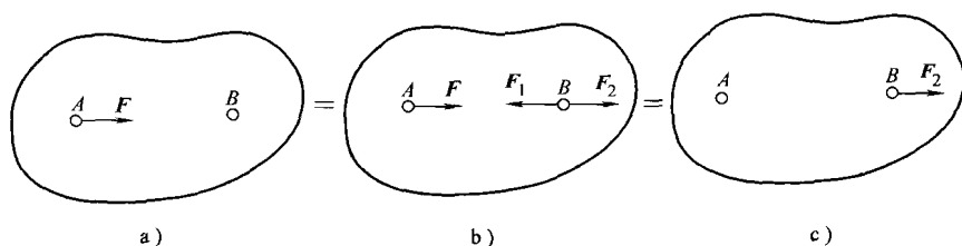
图 1-4 力的可传性原理
