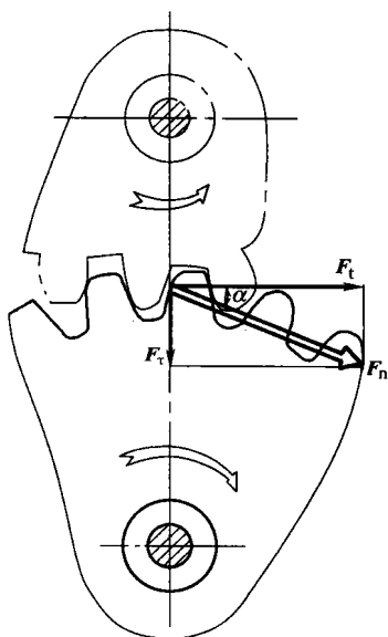
图 1-8 直齿圆柱齿轮受力分析
