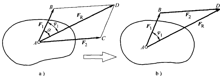
图 1-5 力的平行四边形法则
