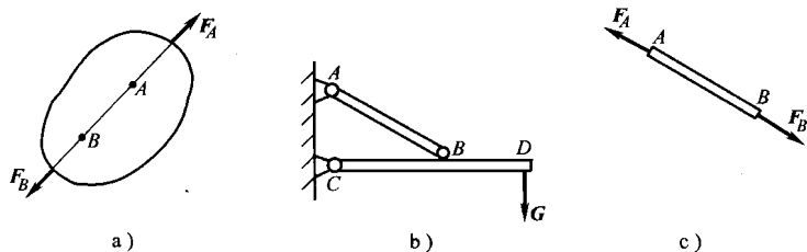
图 1-3 二力构件
