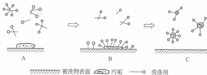
图 2-1 洗涤剂去污原理
