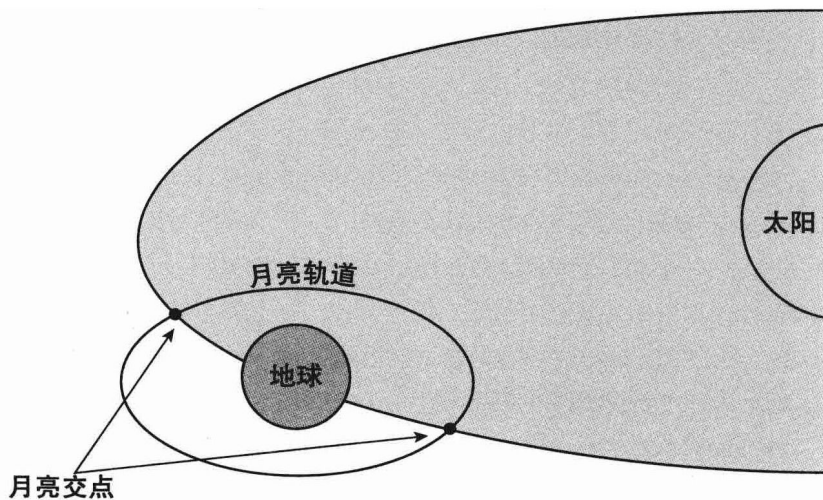
图 1: 从以太阳为中心的角度看月亮交点
