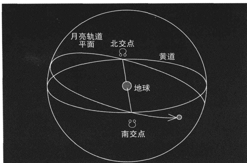
图3：月亮运行穿过地球轨道平面下方的点是南交。月亮穿过地球轨道平面上方的点是北交。
