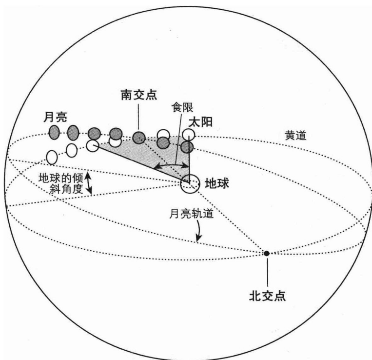
图 2: 在以地球为中心的模型中的日食,表现出和月亮交点连成一线。
