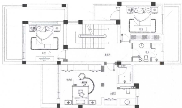
● 二层平面布置图
