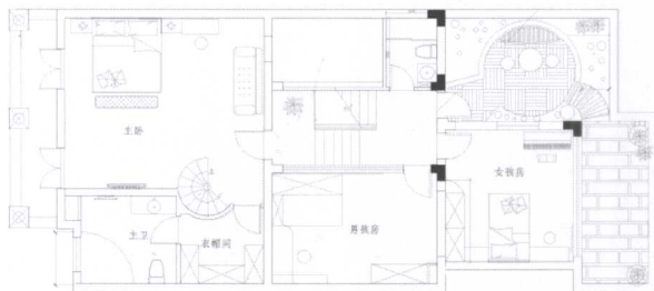
● 三层平面布置图
