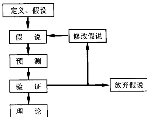
图 1-2 理论的形成
