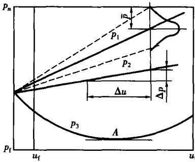
图 1.2 汽车诊断参数随技术状况参数的变化规律
