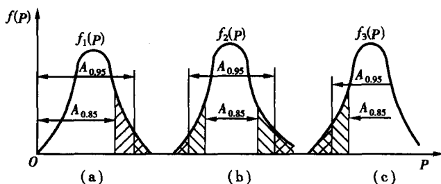
图 1.6 诊断参数标准的确定
