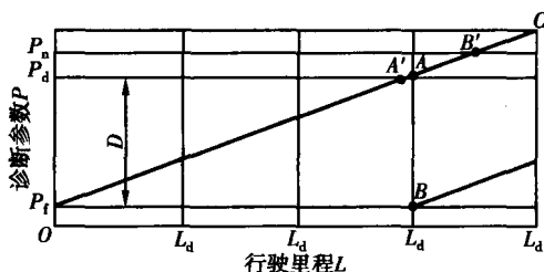
图 1.4 诊断参数随行驶里程的变化情况
