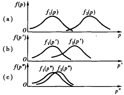
图1.3 诊断参数的信息性
