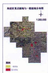
彩插 24-1 海淀区湿地分布图
