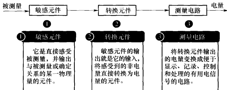
图 1-2 传感器的组成
