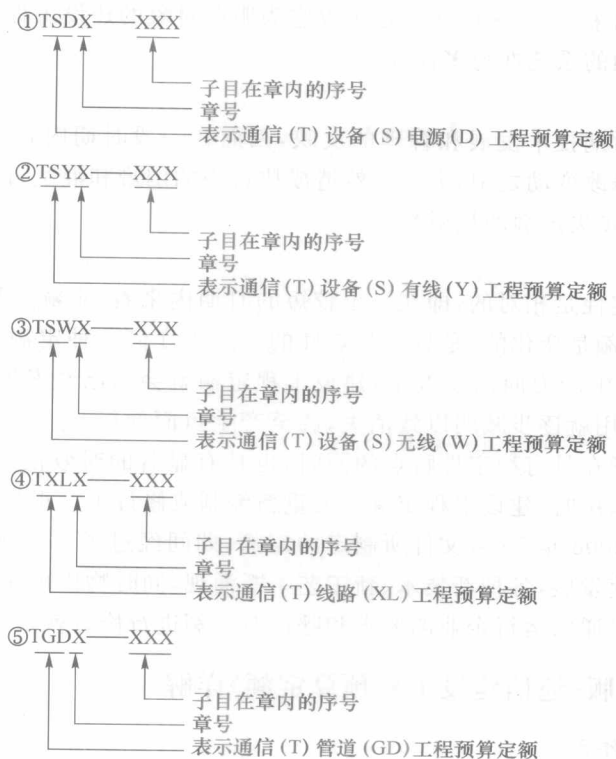
图 2-1 预算定额子目编号示意
